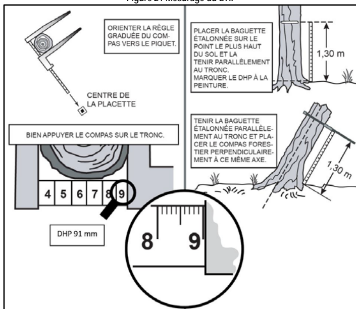
Figure 21 Mesurage du DHP
