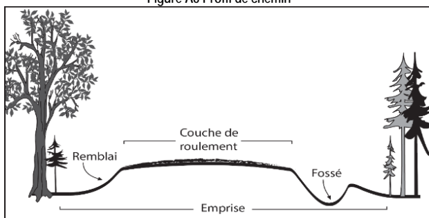
Figure A6 Profil de chemin
