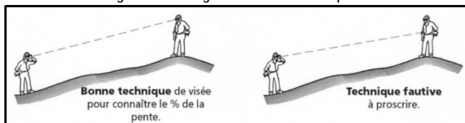
Figure 53 Mesurage de l'inclinaison de la pente
