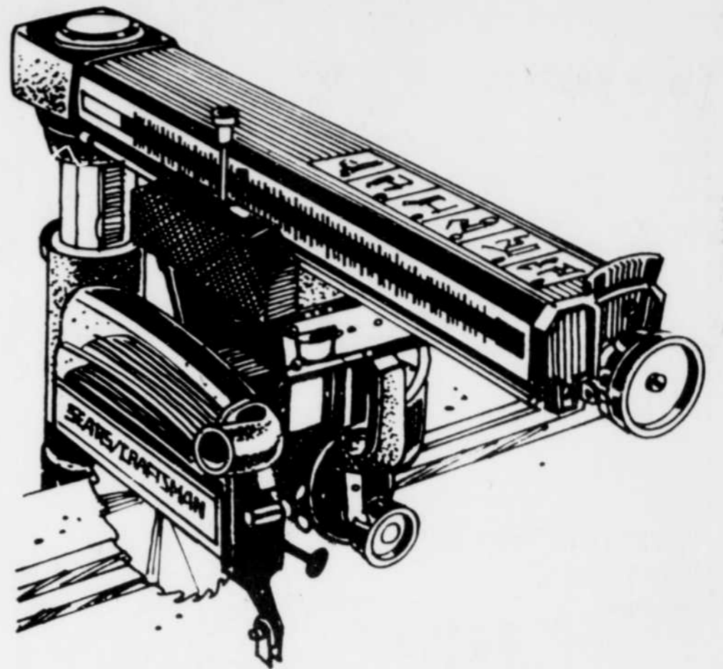
Scie radiale 10"
