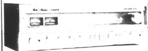
• Recepteur stereo Fisher, modèle RS 1035 AMFM de 35 watts RMS par canal
