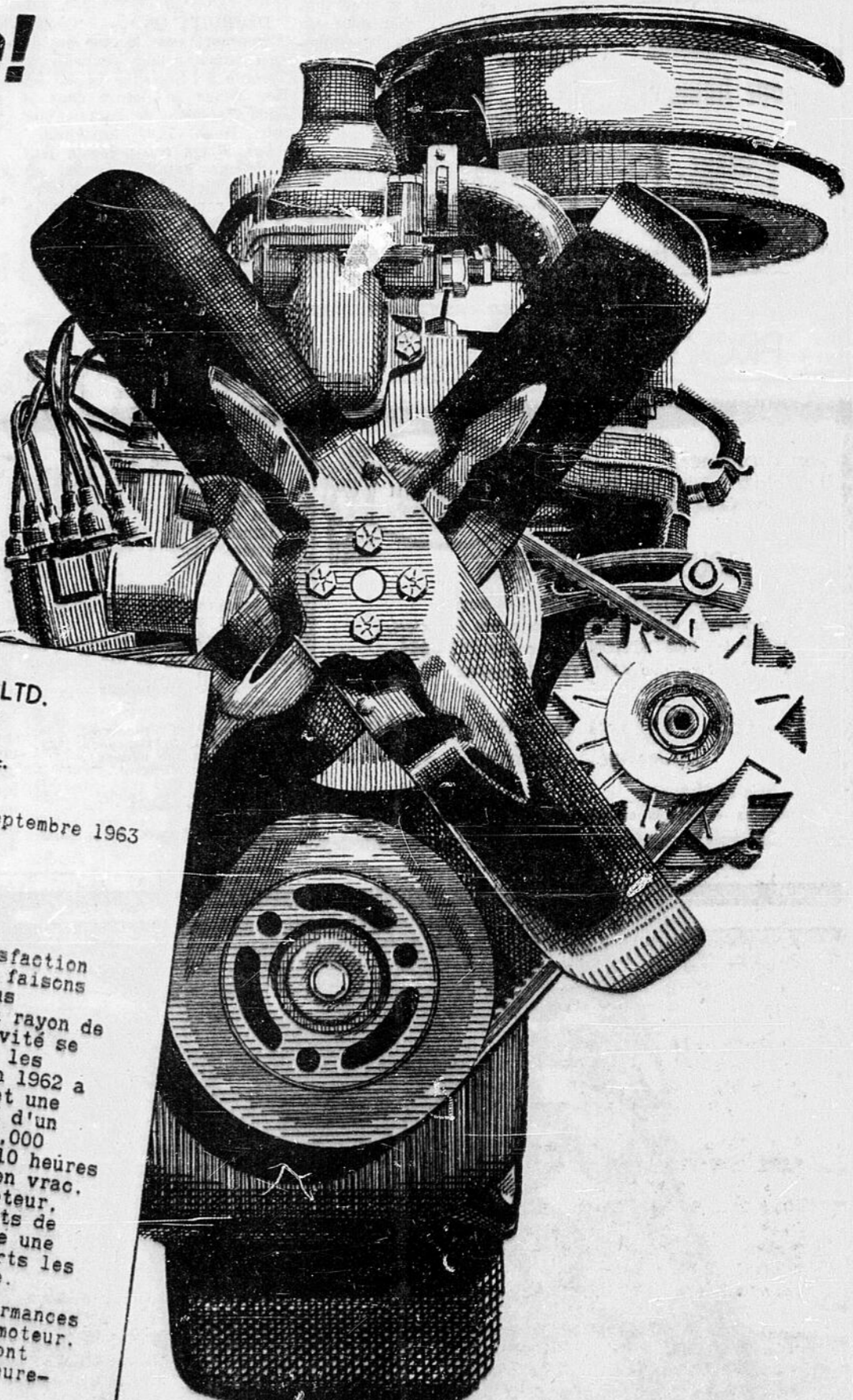
Le six-cyl. 292: un des moteurs de camions 1964, éprouvés à la tâche.
