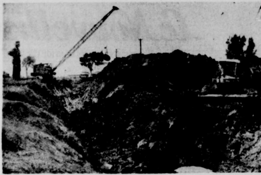
MEME SI LES TRAVAUX proprement dits pour la construction de l'usine de filtration de Louisville ne sont pas encore commencés, les terrains où elle sera édifiée sont actuellement tout bouleversés. Les employés municipaux de Louisville ont entrepris la pose d'un égout pour l'écoulement du terrain qui portera l'édifice. On sait que le conseil de ville et des représentants de l'autorité religieuse se rendront sur les lieux le 28 juillet pour inaugurer officiellement les travaux.
