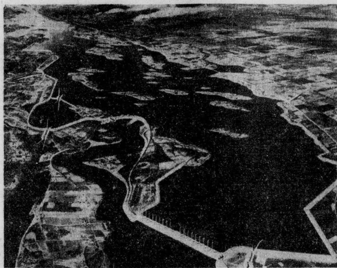
LA CANALISATION DU ST-LAURENT: Ce dessin, publié par FRANCIS-B. WILBY, président de la Commission hydraulique de l'Etat de New-York, a été préparé d'après les plans des ingénieurs du projet de canalisation du St-Laurent. Il donne une vue d'ensemble du projet une fois qu'il sera terminé. Le projet général prévoit la construction d'une centrale électrique de 2.200.000 chevaux-vapeur près de Massena, N.-Y., dans la section d'a Rapides Internationaux, et d'une voie navigable pour les océaniques jusqu'aux Grands Lacs. La profondeur requise du chenal, 27 pieds, existe déjà sur environ 90 pour cent du parcours, allant de Duluth-Chicago jusqu'à la mer. Le Canada a déjà dépensé $132.672.000 et les Etats-Unis, 631.742.000, pour des travaux formant partie intégrale du projet actuellement devant le Congrès. La plus grande partie des travaux qui restent à accomplir sont dans la section des Rapides Internationaux. Ce dessin illustre les principaux travaux projetés dans cette section. A droite, en bas, la centrale de Barghant Island, qui aura une capacité de 2.200.000 c.v. Au centre, la digue du Long Sault et, à gauche, les écluses devant servir à la voie maritime. (Central Press)
