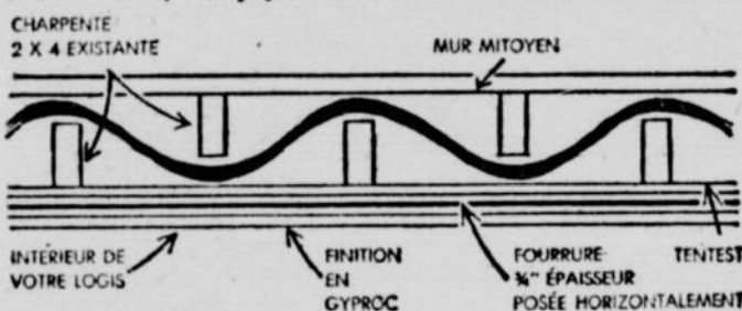
Plan d'un mur mitoyen avec insonorisation
