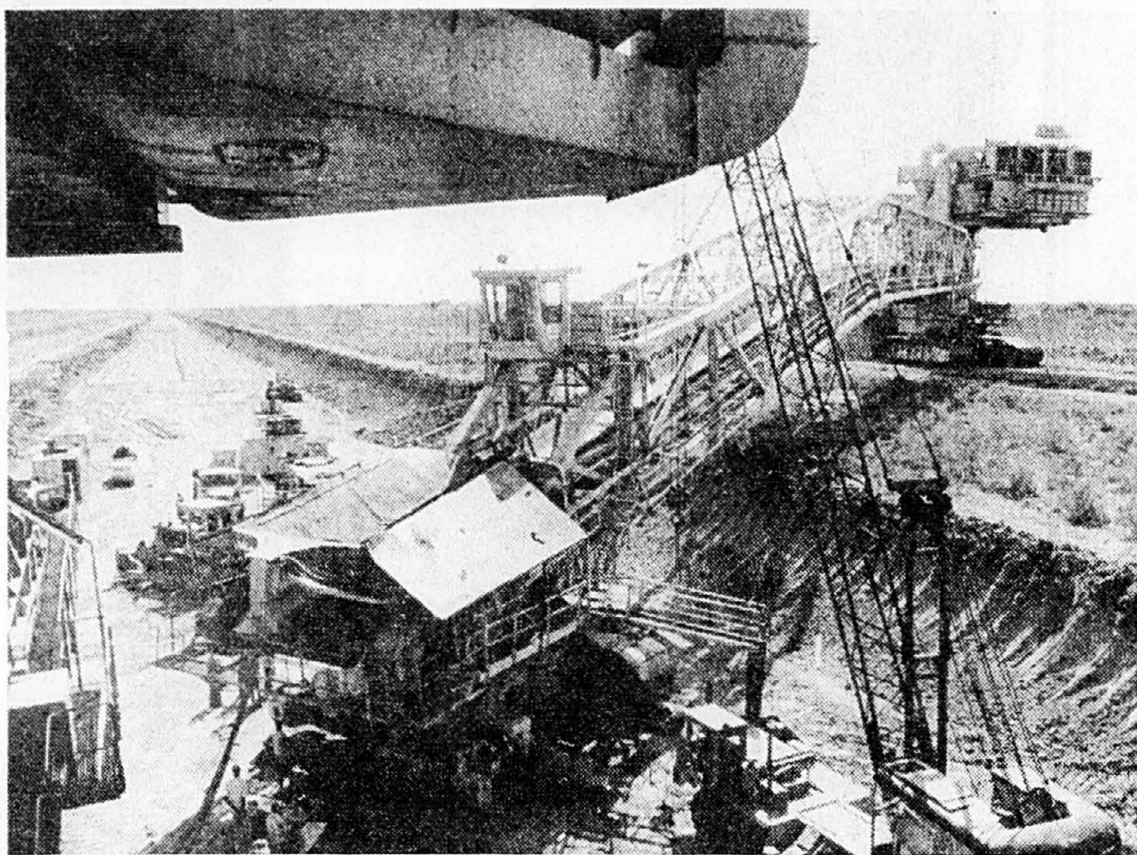
Les travaux du canal de Jonglei, le plus grand chantier d'Afrique.
