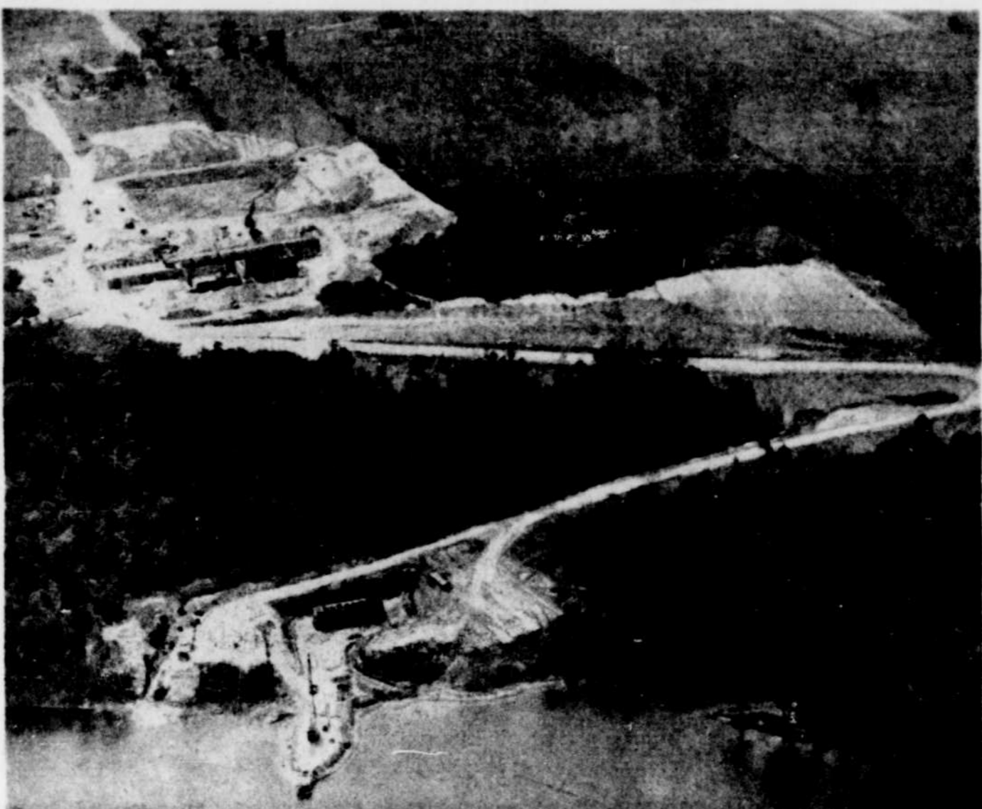
CETTE VUE AERIENNE montre parfaitement que les travaux de construction des quatre parties de l'usine: conduite d'aménée, usine de pompage, usine de filtration et réservoir sont menés à peu près de pair.
