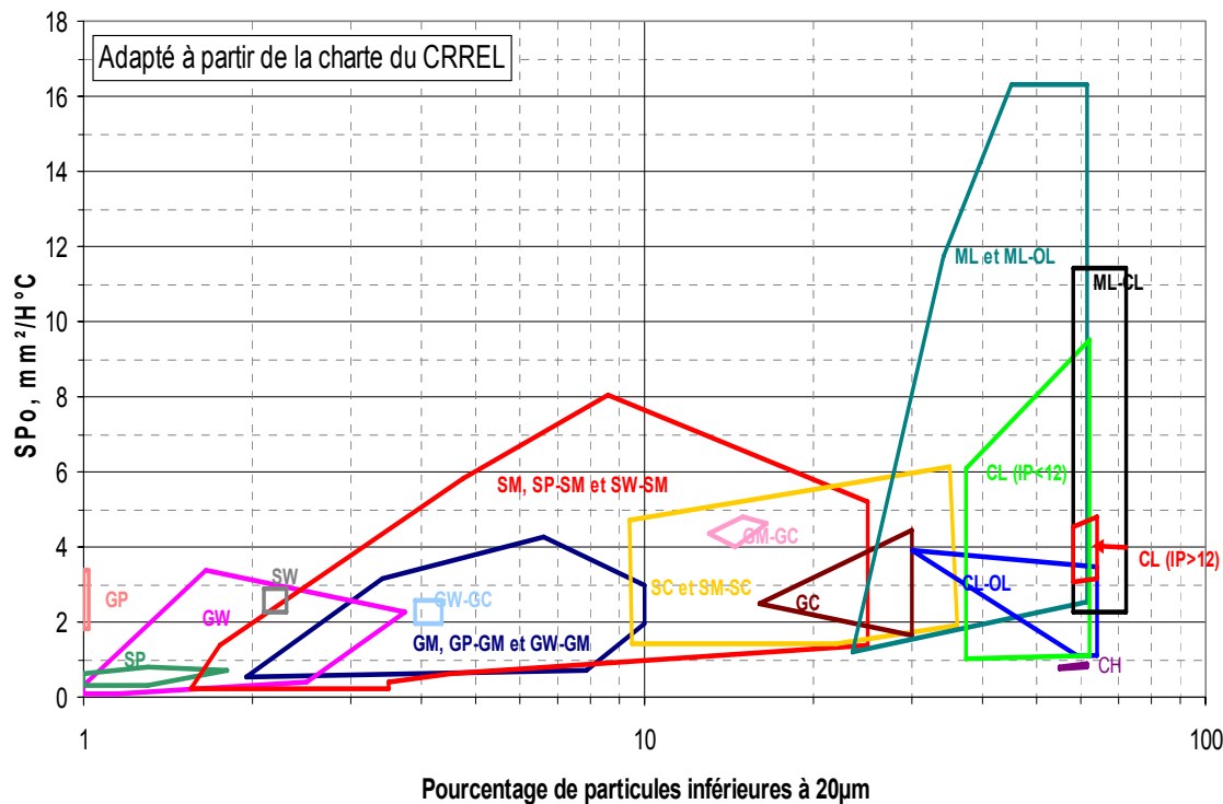
Figure 8 : Charte du CRREL convertie pour l'indice SP 0
