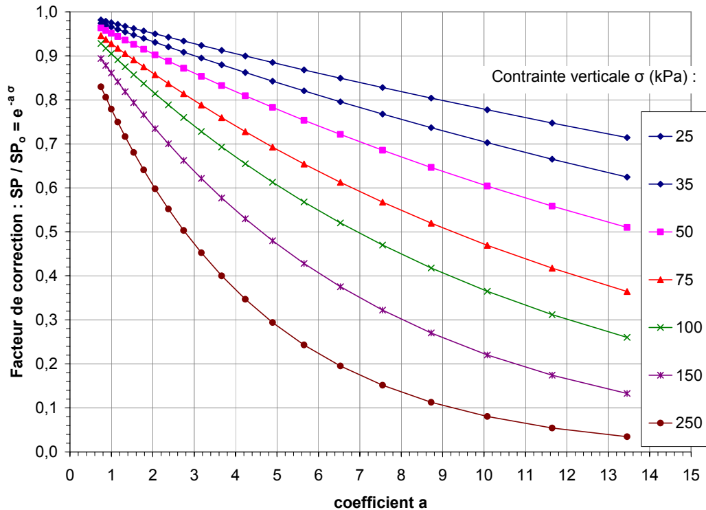
Figure 12 : Effet du coefficient de surcharge sur la gélivité
