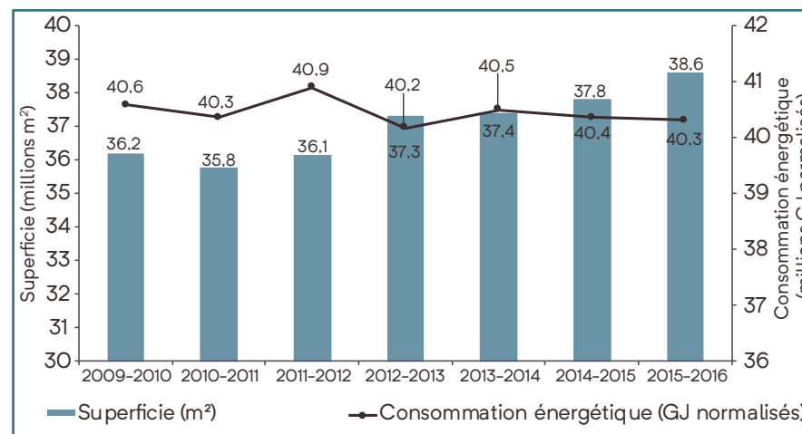
Figure 3 Évolution de la superficie et de la consommation énergétique normalisée des bâtiments publics, de 2009-2010 à 2015-2016
