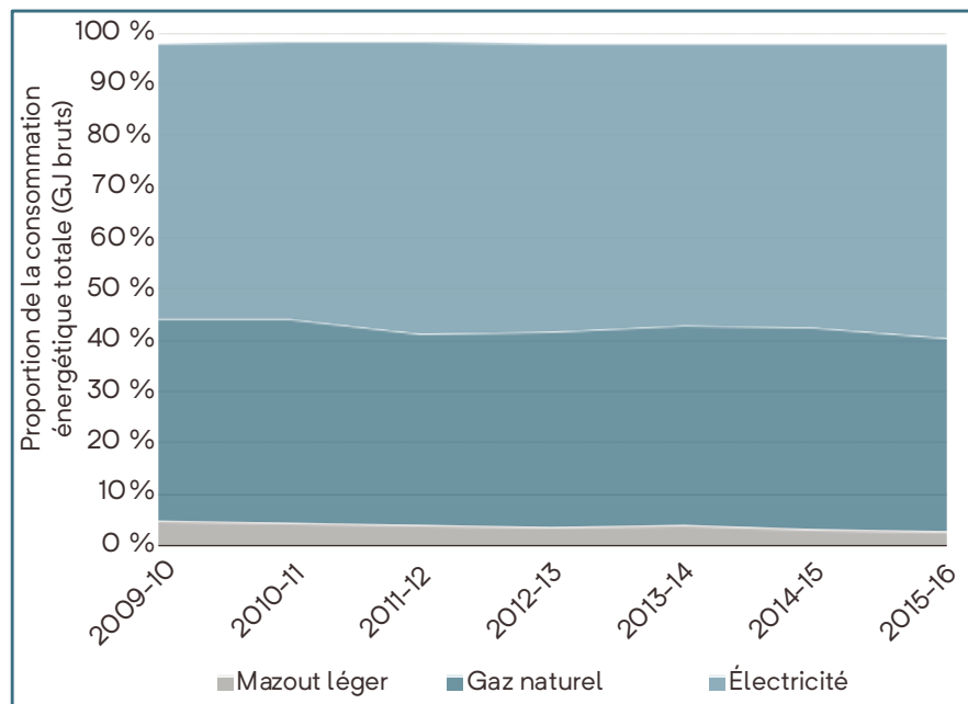
Figure 4 Évolution des proportions des principales formes d'énergies consommées dans les bâtiments publics (électricité, gaz naturel, mazout léger) entre 2009-2010 et 2015-2016
