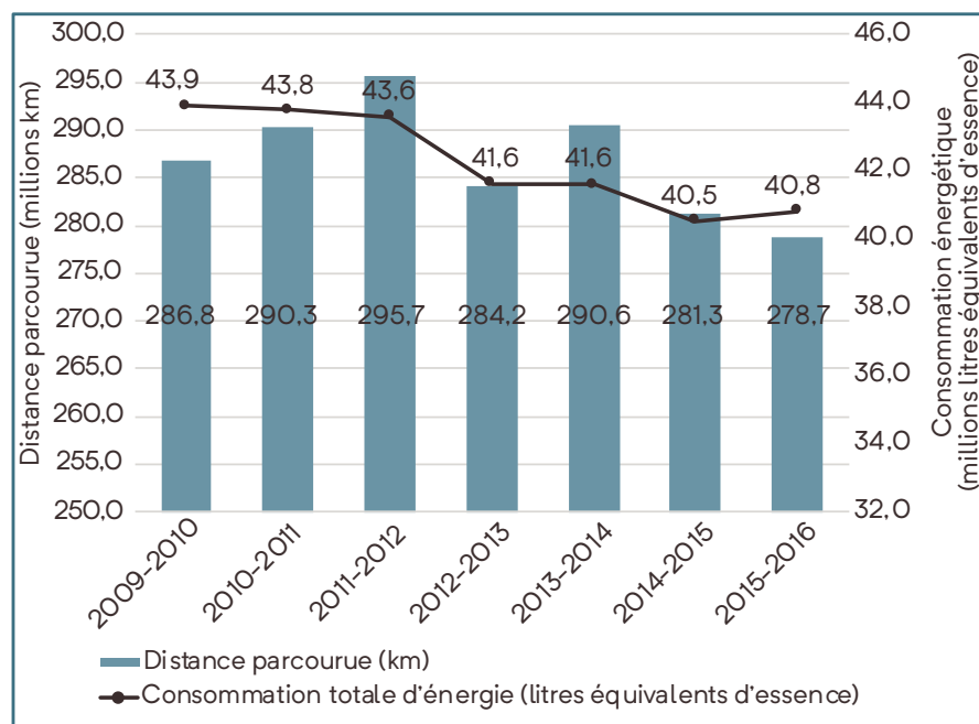
Figure 7 Évolution de la distance parcourue (km) et de la consommation énergétique (litres équivalents d'essence), de 2009-2010 à 2015-2016
