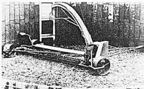
DÉCHARGEUR AUTOMATIQUE POUR 1... 2... 3 SILOS OU PLUS
