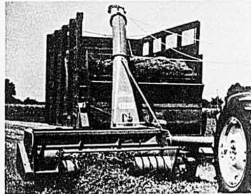
Pour hacher le fourrage: l'étonnante récolteuse Ford 612 hache aussi bien les ensilages sarclés et les ensilages verts. Elle s'adapte en quelques minutes à n'importe quel type de hachage et offre à la fois haut rendement et économie.
