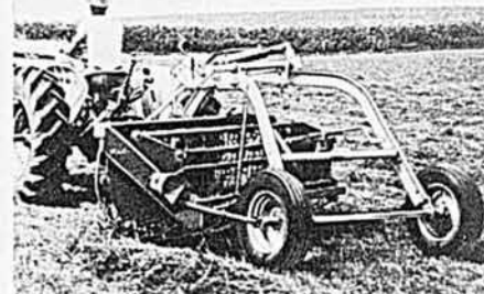
RATEAU CASE 281 À DÉCHARGE LATÉRALE—ramasse un andain de 8' 4" à une vitesse allant jusqu'à 7 m.p.h. Nettoie parfaitement les terrains accidentés.
