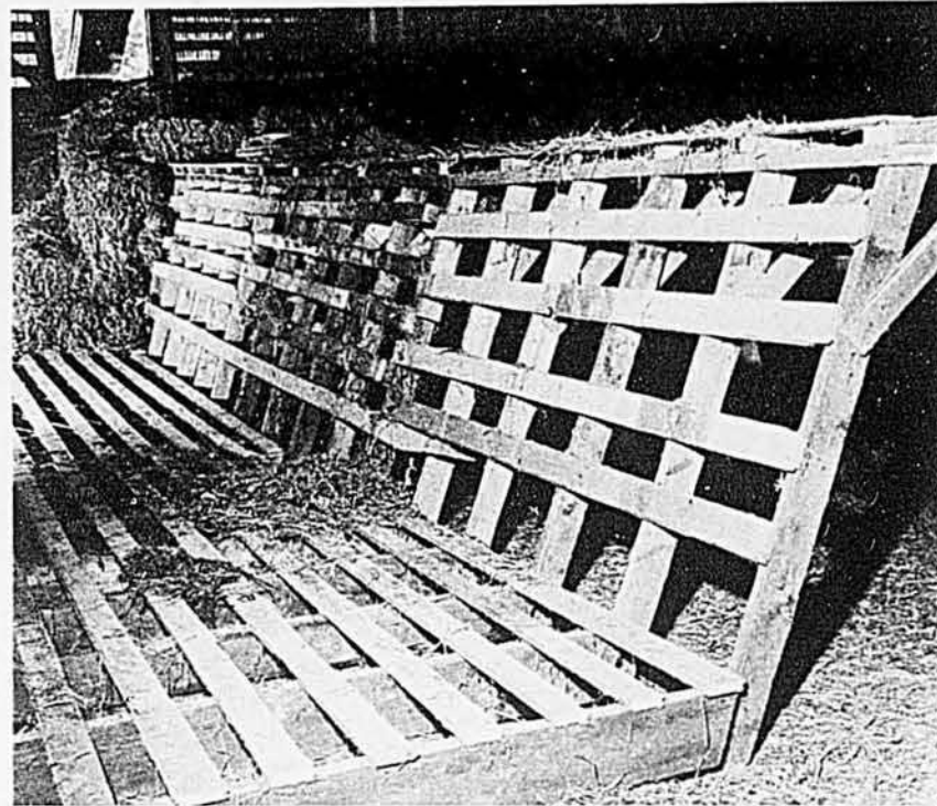
Le séchage artificiel du foin est peut-être la solution au problème. Il permet d'enranger un foin dont le pourcentage d'humidité est encore beaucoup trop élevé. On le voit ici, l'organisation est simple, de l'air, chauffé ou non, est tout simplement poussé avec pression sous ce plancher ajouré qui a été fait de vieux bois.
