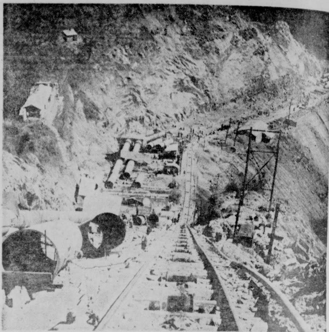
Cette photographie donne une idée de l'ampleur des travaux du projet hydro-électrique de Kundah. Ces tuyaux installés sur une très forte pente font subir un bond considérable aux eaux qui alimenteront plus bas une centrale électrique. D'ailleurs, la photo permet de voir parfaitement bien l'angle de la pente et la nature du terrain où s'effectuent les travaux. A droite, on distingue les rails servant à hisser les tuyaux.
