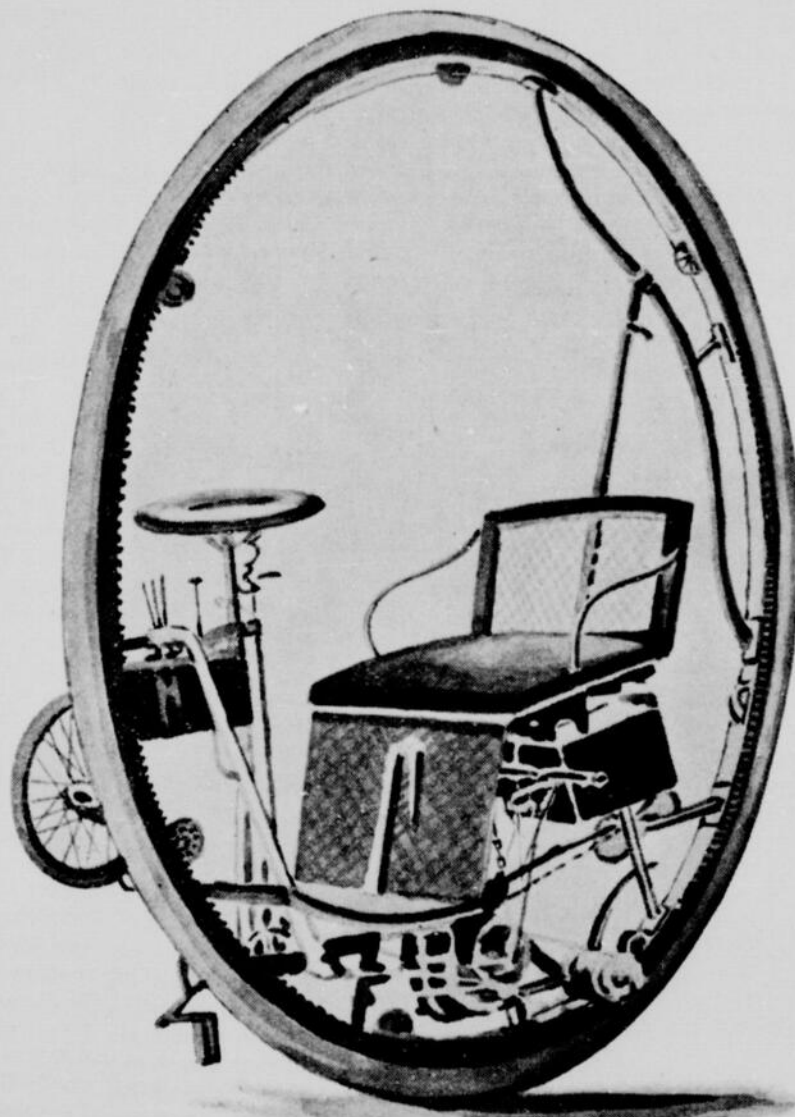
L'automobile monocycle
