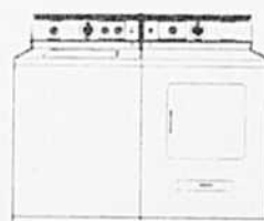
Modèle "SPATIAL"
