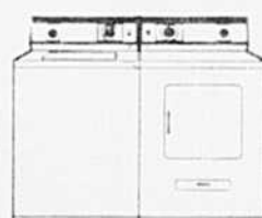
Modèle "SATELLITE"
