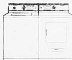
Modèle "COSMOS"
