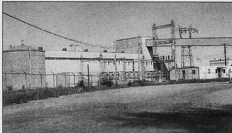
Boralex brûle la biomasse des scieries pour chauffer de l'eau destinée à produire de la vapeur à très haute pression qui fait tourner une turbine et crée de l'électricité pour Hydro-Québec.
