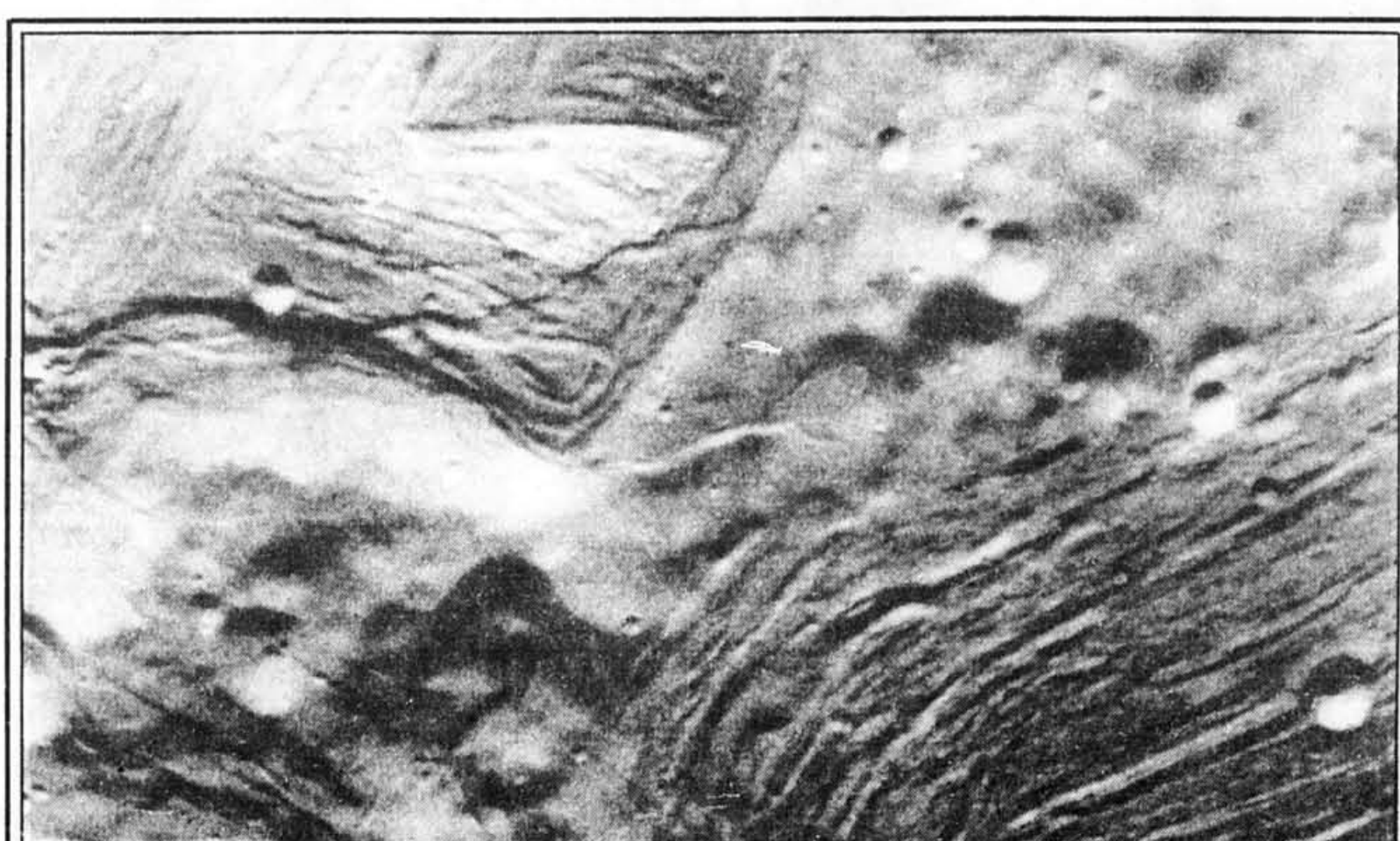
Le relief extraordinaire de Miranda intrigue au plus haut point les chercheurs du Jet Propulsion Laboratory de Pasadena.
