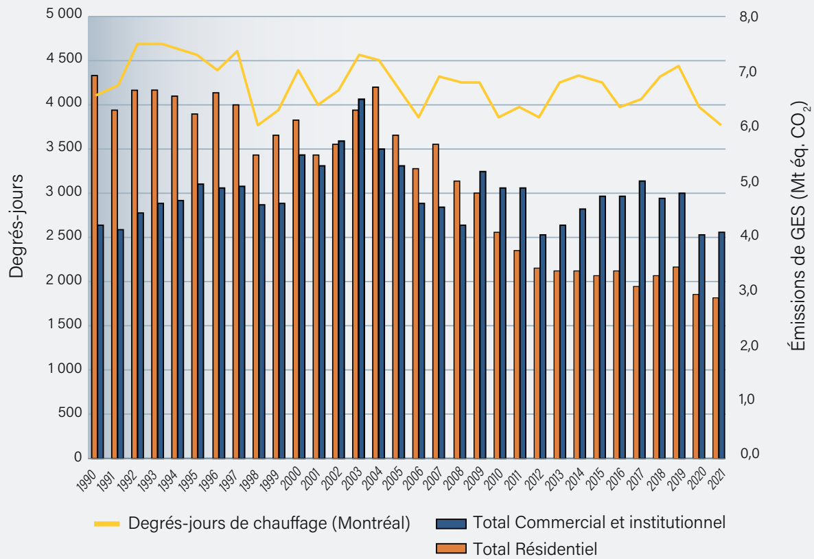
Figure 21 Fluctuation des émissions de GES des sous-secteurs « résidentiel » et « commercial et institutionnel » et des degrés-jours de chauffage (CANADA, 2023) 7 de 1990 à 2021
