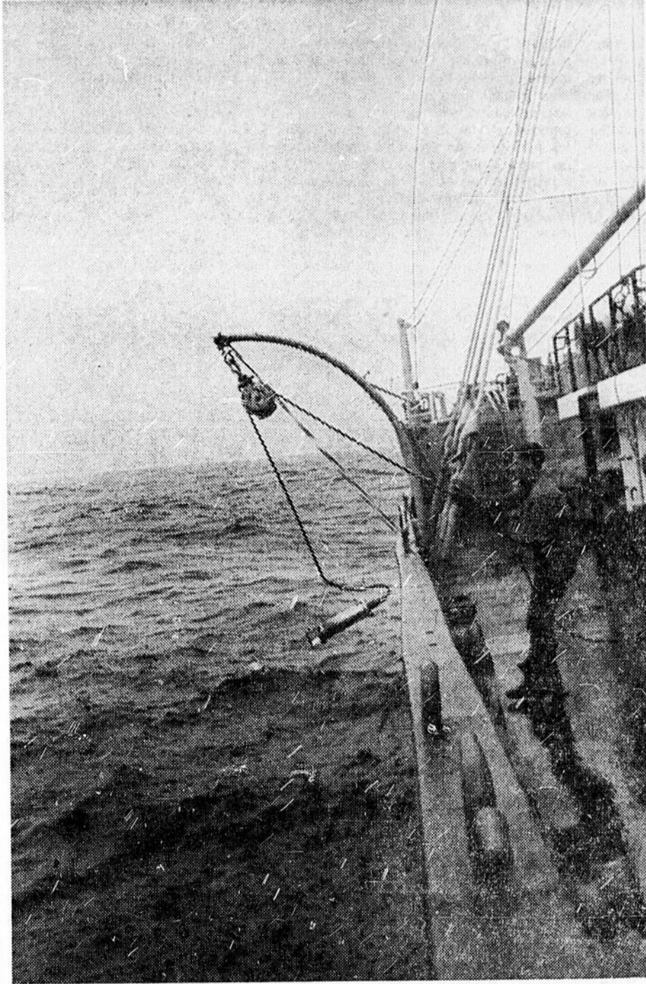
Un bathythermograhe électronique est descendu le long du M. V. Martin Karlsen, un vaisseau nolisé et orienté vers la recherche scientifique au Centre canadien des eaux intérieures à Burlington, en Ontario.
