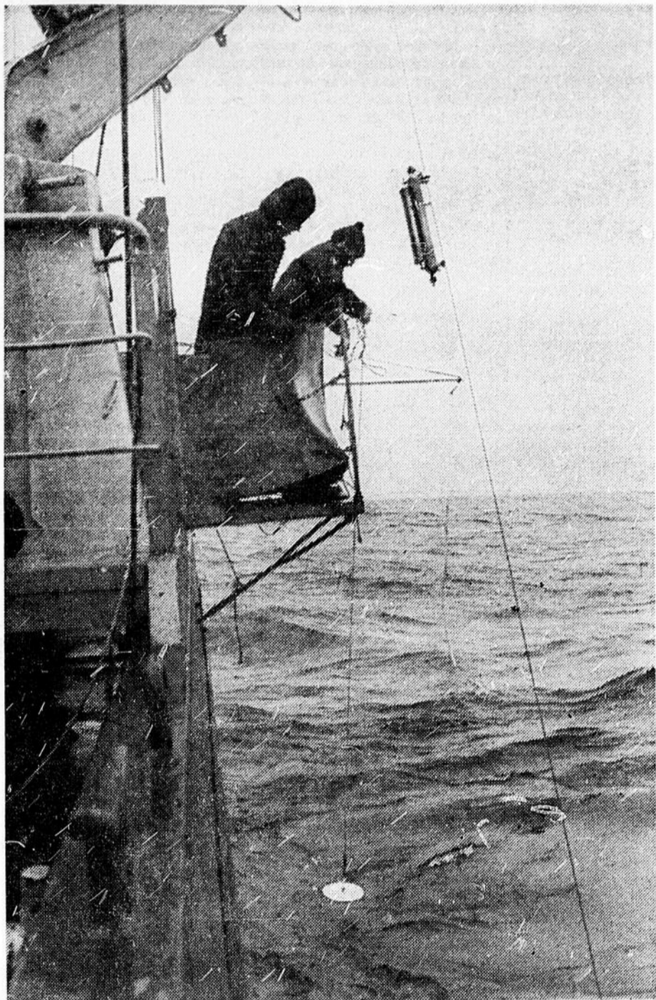
UNE BOUTEILLE BASCULANTE, dite Knudsen, est immergée dans l'eau pour y enregistrer des températures et y prendre des échantillons d'eau tandis qu'un disque dit secchi est également déposé à l'eau pour y mesurer la transparence.
