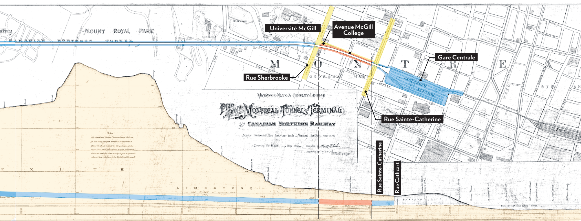
Vue en plan et profil du tunnel du mont Royal. Source: AMT
