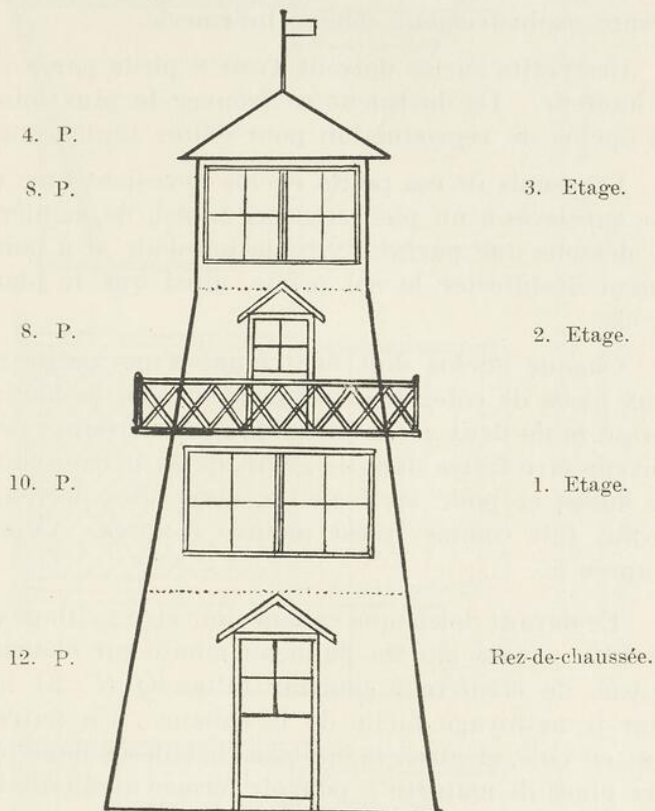
TOUR D'OBSERVATION, ENTREE ORIENTEE AU SUD.
