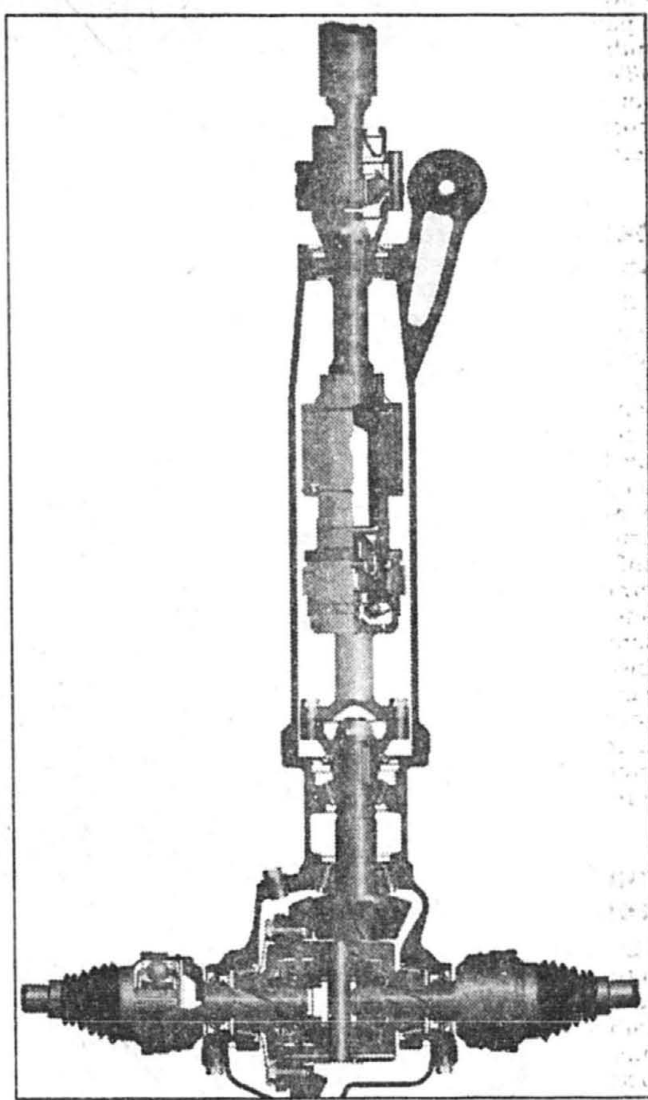
La partie centrale du système de traction de Volvo abrite le viscosoupleur et le système de roue libre, deux éléments intégrés dans un tube de couple pour plus de rigidité.
