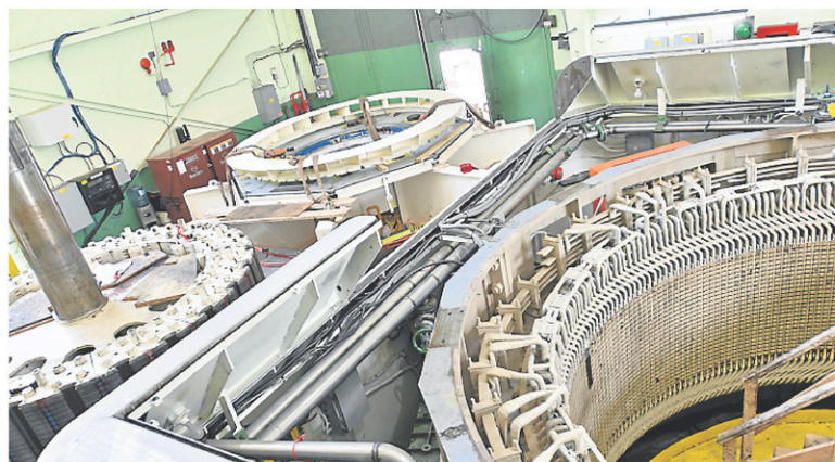
La roue d'eau principale de la centrale Jim-Gray sera remplacée d'ici octobre.
