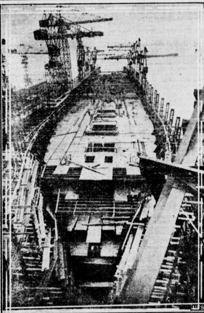
Cette photo nous montre le futur paquebot de la ligne Cunard-White Star qui sera baptisé "Mauretania", et qui est actuellement en construction à Birkenhead, Angleterre. Il aura 750 pieds de longueur et sera plus large que le premier "Mauretania" qui, durant 22 ans fut le plus rapide paquebot de l'Atlantique.
