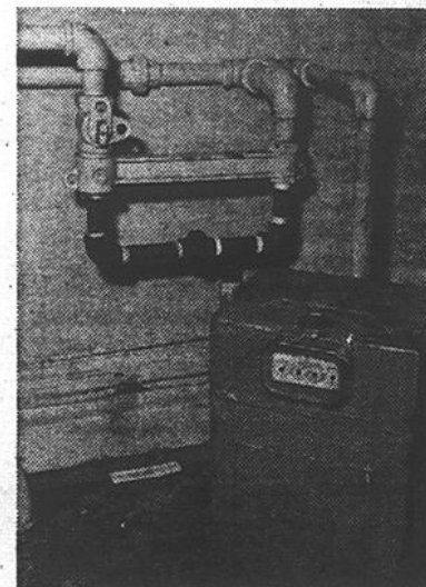
Voilà: l'ouvrage est terminé. Le compteur est désormais inutile, et le gaz coule à flots dans les tuyaux, à l'insu de la compagnie. Durée de l'opération: un quart d'heure. C'est propre, gratuit, et absolument illégal. Il ne reste plus qu'à vérifier que tous les "pilotes" de tous les appareils sont allumés, et la maison se retrouve à nouveau chauffée, munie d'un poêle et d'un réservoir à eau chaude qui fonctionnent...
