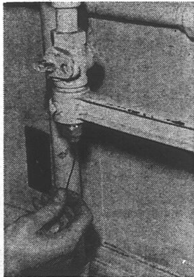
Le sceau du bas, qui obstrue le tuyau d'alimentation, est un simple boulon qui tourne à vide. Pour parvenir à le dévisser, on y introduit une tige de métal (un hameçon no 16 redressé à la chaleur) pour en faire bouger les mécanismes intérieurs, jusqu'à ce que ceux-ci s'enclenchent, et que le boulon se dévisse comme n'importe quelle "belle" normale.
