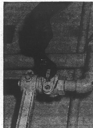
Il ne reste plus qu'à rétablir le "circuit" du gaz en déplaçant la valve en position "ouverte" à l'aide d'une clef à molette, après s'être assuré que tous les appareils fonctionnant au gaz sont proprement branchés, pour éviter une éventuelle (et catastrophique) fuite.
