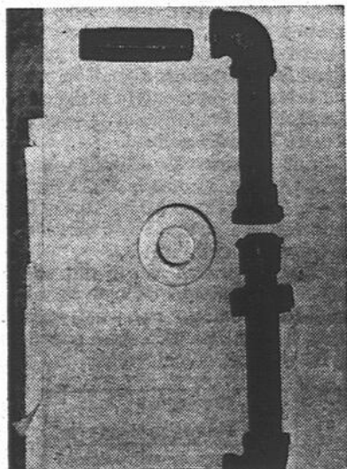
Quatre bouts de tuyau de fer noir (celui qu'utilisent des employés de Gaz Métropolitain), quatre jointures, et du ruban isolant de Teflon: c'est tout ce qu'il faut pour remplacer un compteur.
