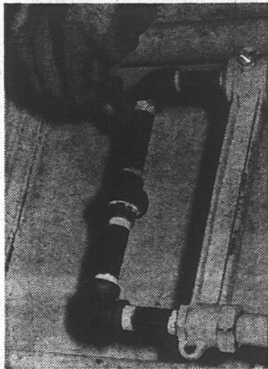
Les tuyaux sont mis en place et ajustés avec soin. Toutes les jointures sont isolées avec du ruban Teflon; on vérifie l'étanchéité de l'ensemble... avec du savon à vaisselle, qui se gonfle et fera une bulle à la plus petite fuite. Les employés du Gaz utilisent, soit un détecteur de gaz, soit un "savon spécial" très semblable au savon à vaisselle.
