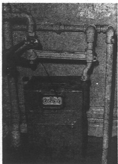
Le compteur à gaz n'a d'autre utilité que d'enregistrer le nombre de pieds cubes de gaz consommé. Le gaz arrive par le tuyau de gauche, passe par le compteur, en ressort par le tuyau de droite, pour être distribué aux différents appareils domestiques. Quand ils viennent "couper", les employés de Gaz Métropolitain ferment une valve, et en bloquant le fonctionnement par un sceau spécial (celui du haut) puis débranchent le tuyau d'alimentation du compteur, et bloquent ce tuyau par un second sceau, celui du bas.
