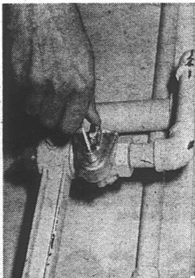
Une valve de gaz est ouverte quand elle est placée dans le sens de la tuyauterie, et fermée quand elle est placée en travers, comme dans la photo ci-haut. À l'aide d'une mince tige de plastique, le "pirate du gaz" fait jouer les petits boulons, qui retiennent le sceau en position fermée, jusqu'à ce que le mécanisme se déclenche.
