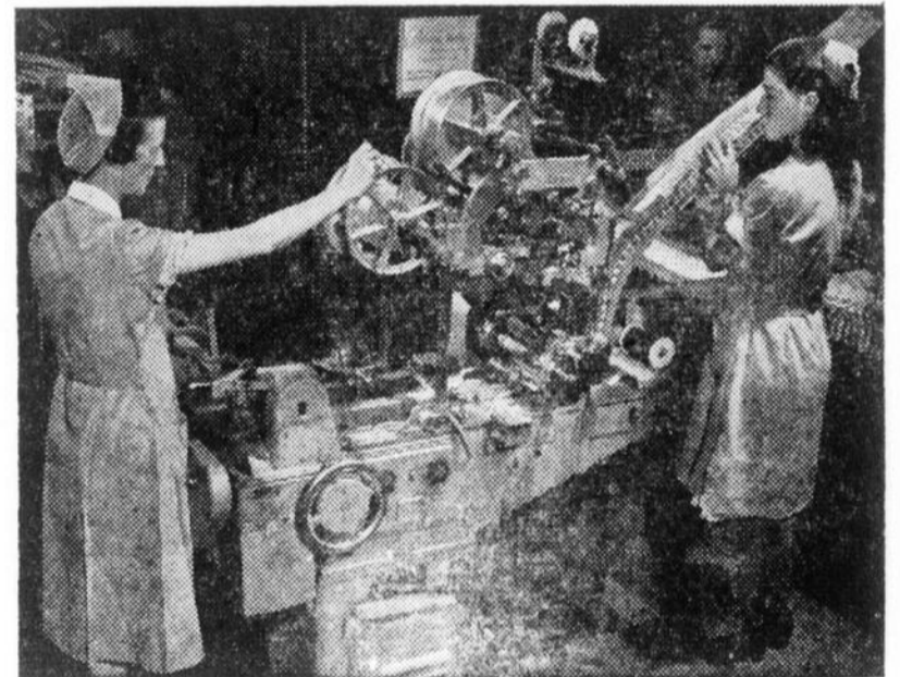
Cet appareil enveloppe dans la pellicule cellulosique "Cellophane" quelque 200 paquets de cigarettes à la minute. Le Canada suffit à presque 98 pour cent de sa consommation de tabac, alors qu'en 1930, il en importait près de 60 pour cent.
