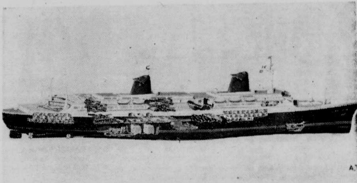
Le nouveau paquebot de la Compagnie French Line. Nom "FRANCE" sera lancé le 11 mai 1960. Construit par les Chantiers Penhoet de St-Nazaire. Long. 1,000 pieds. Larg. 100 pieds. Creux 75 pieds. Tirant d'eau 30 pieds. Déplacement en charge 55,000 tonnes. Vitesse 30 nœuds. Puissance 150,000 C.V. Passagers 2,000. 4 hélices. 2 picines. Garage pour 100 voitures. Cinéma 600 personnes. Ligne en service. Le Havre-New-York.
