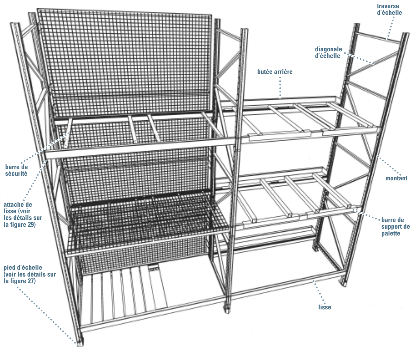
Figure 26. Composants et accessoires de palettier (Illustration : Technirack)
