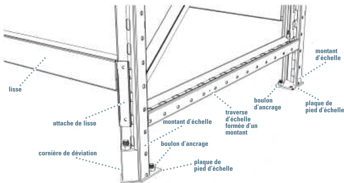
Figure 42. Protection intégrée aux montants (Illustration : Technirack)
