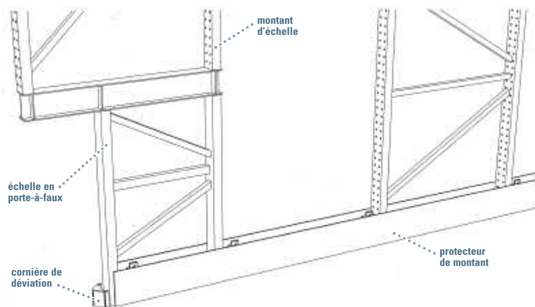
Figure 30. Échelle en porte-à-faux
