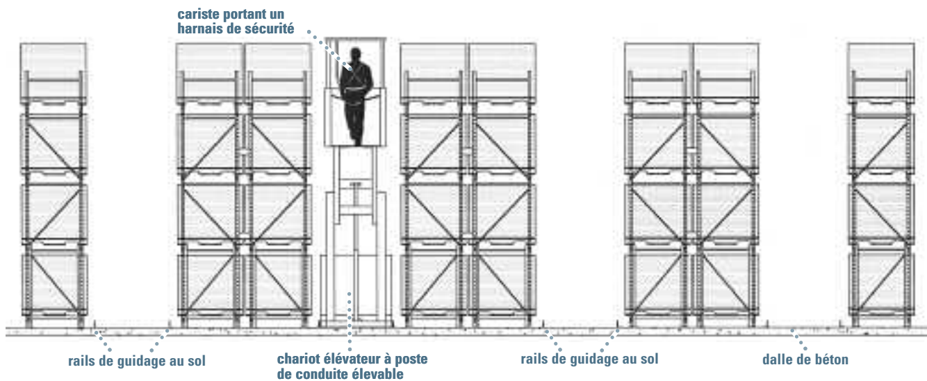
Figure 46. Allée de service très étroite et chariot élévateur à poste de conduite élevable (Illustration : Technirack)
