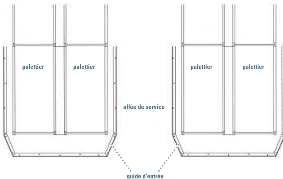
Figure 48. Guide d'entrée (Vue de plan)
