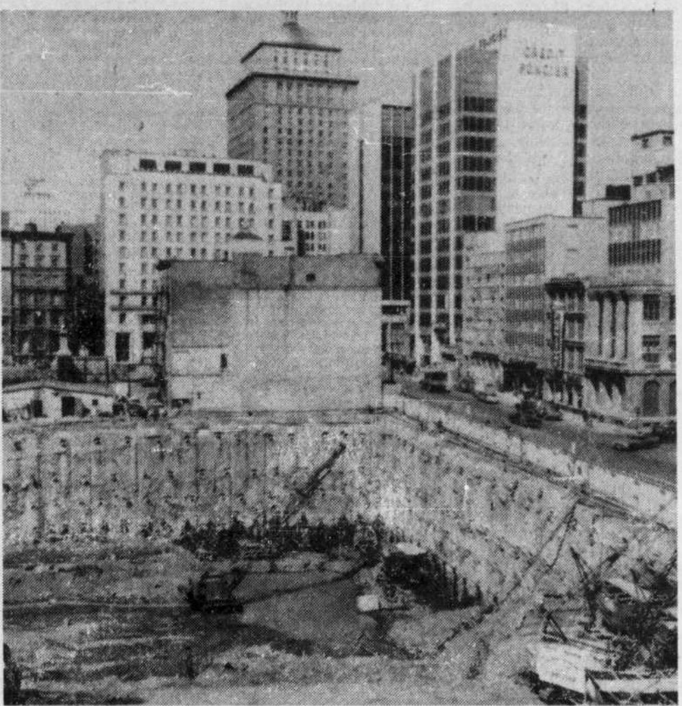
Des travaux de forage sont en cours pour le mur-diaphragme qui borde le terrassement du gratte-ciel Place Victoria de 48 étages qui s'élèvera à Montréal, et dont l'achèvement est prévu pour 1967. L'entrepreneur classique entraîne la pose interne de moises, et il en résulte une surface de travail restreinte au cours de la construction. Cependant, un mur-diaphragme maintenu en place par des câbles en acier servant de haubans assure de grands espaces libres. Les câbles sont ancrés dans la masse du roc après le percage de trous à des angles de 45 degrés dans le terrain de recouvrement. Plus de 450 trous de quatre pouces de diamètre et ayant jusqu'à 120 pieds de long étaient terminés le 15 juin.
