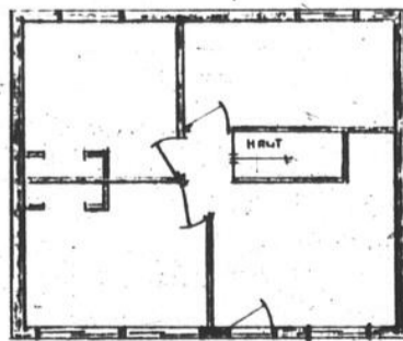
PLANCHER DE FONDATION PROPOSÉ (25' x 21')
