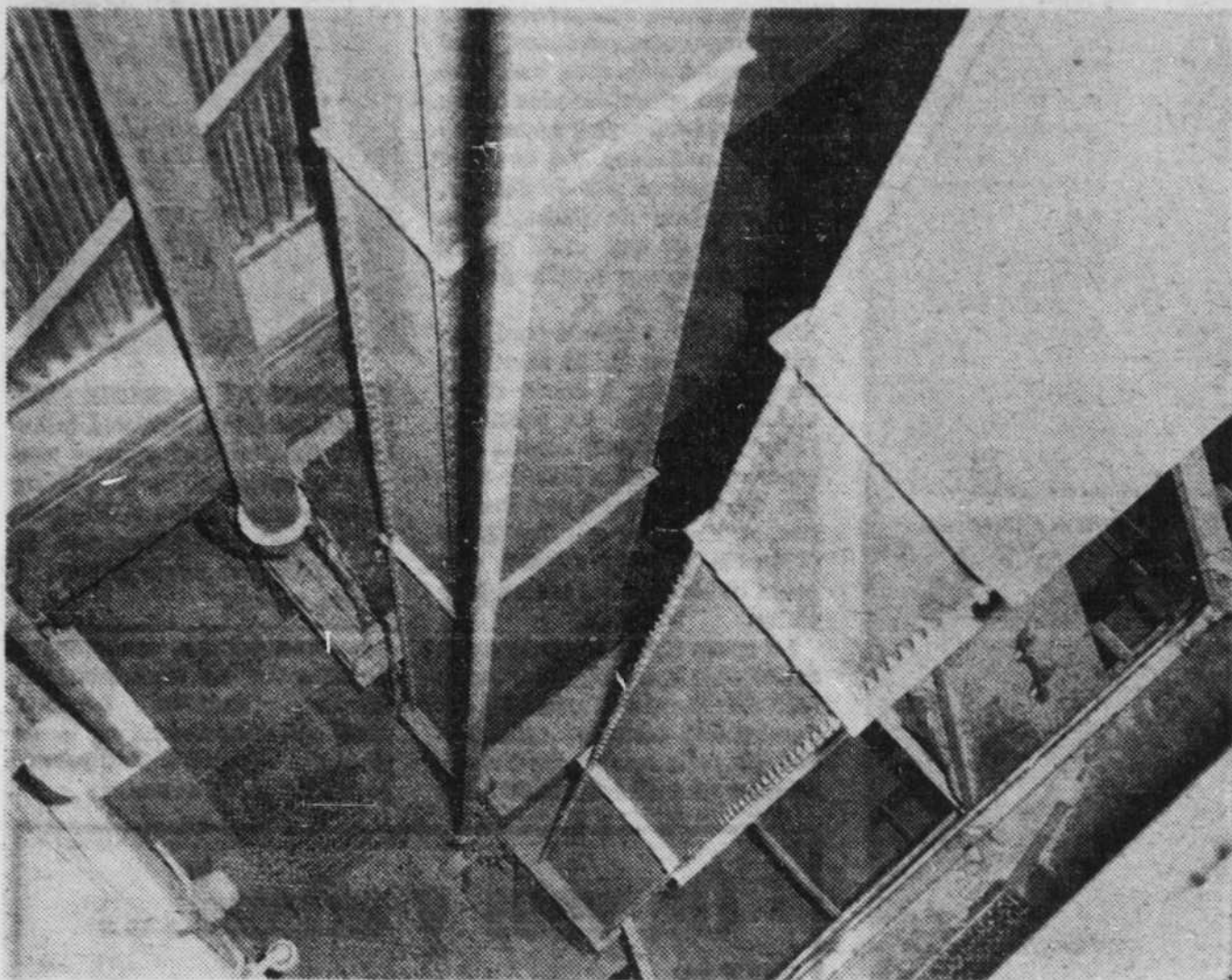
SAGUENAY TERMINALS à Port-Alfred est un exemple typique des quantités d'aluminium de plus en plus grandes qu'on utilise aujourd'hui pour les immeubles et même pour l'équipement des installations maritimes. Ci-dessus, vue en plongée d'un élévateur d'alumine, au quai Duncan.
