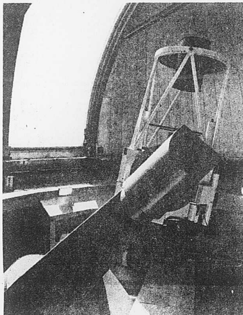
Le télescope de l'Observatoire astronomique du Québec pointe ici vers le ciel par la baie d'observation qui mesure 15 mètres de longueur et 3 mètres et demi de largeur. Pour éviter toute vibration qui dérangerait l'ajustement de l'instrument, le soc et les câbles électriques du télescope sont indépendants de la structure même de l'observatoire.
