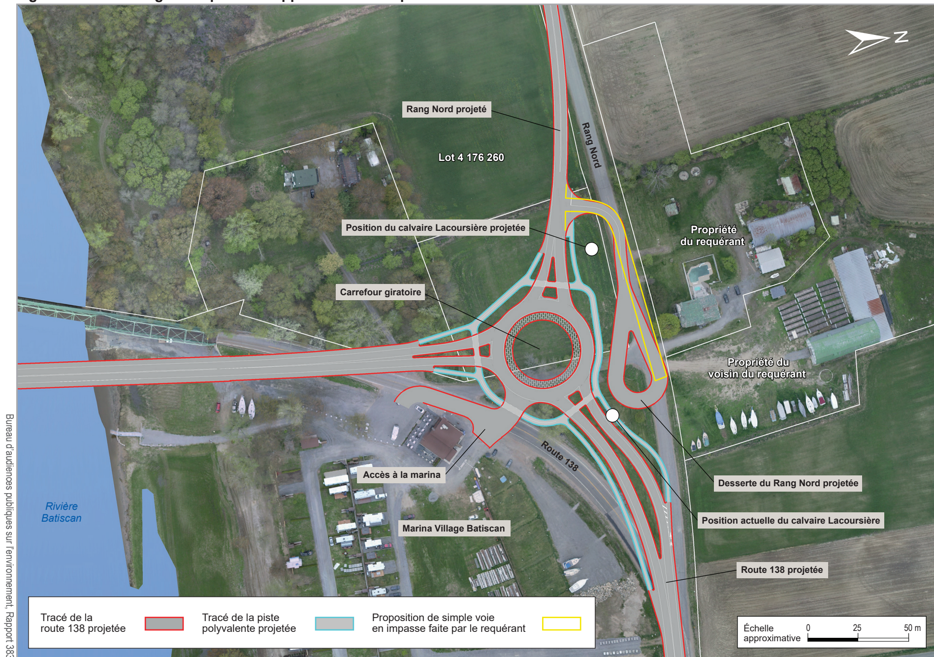
Figure 2.4 L'aménagement prévu à l'approche nord du pont
