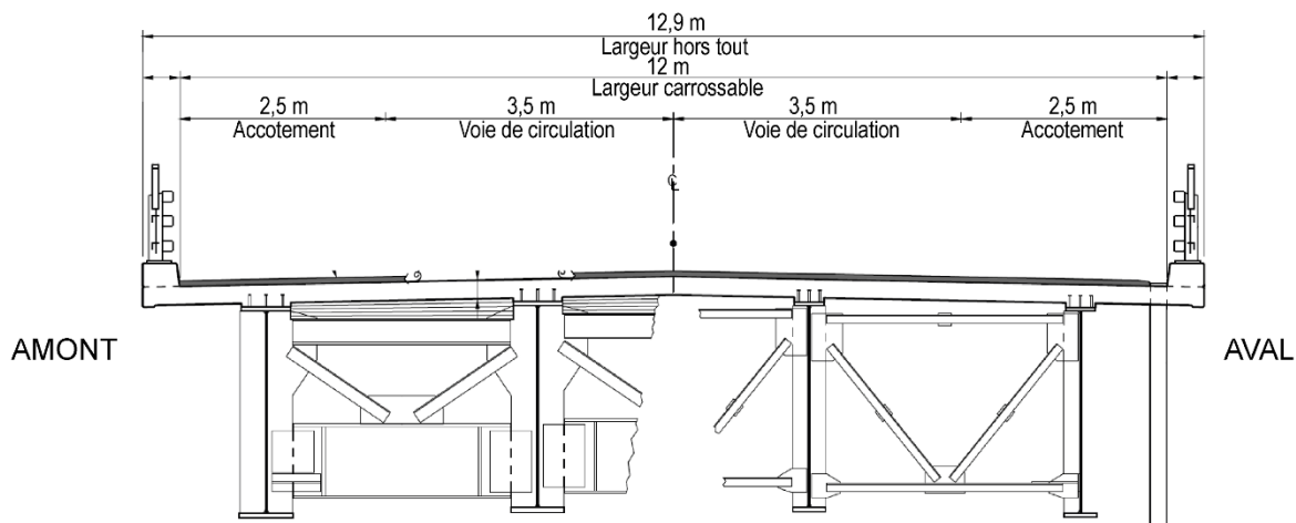
Figure 2.3 La coupe transversale du pont
