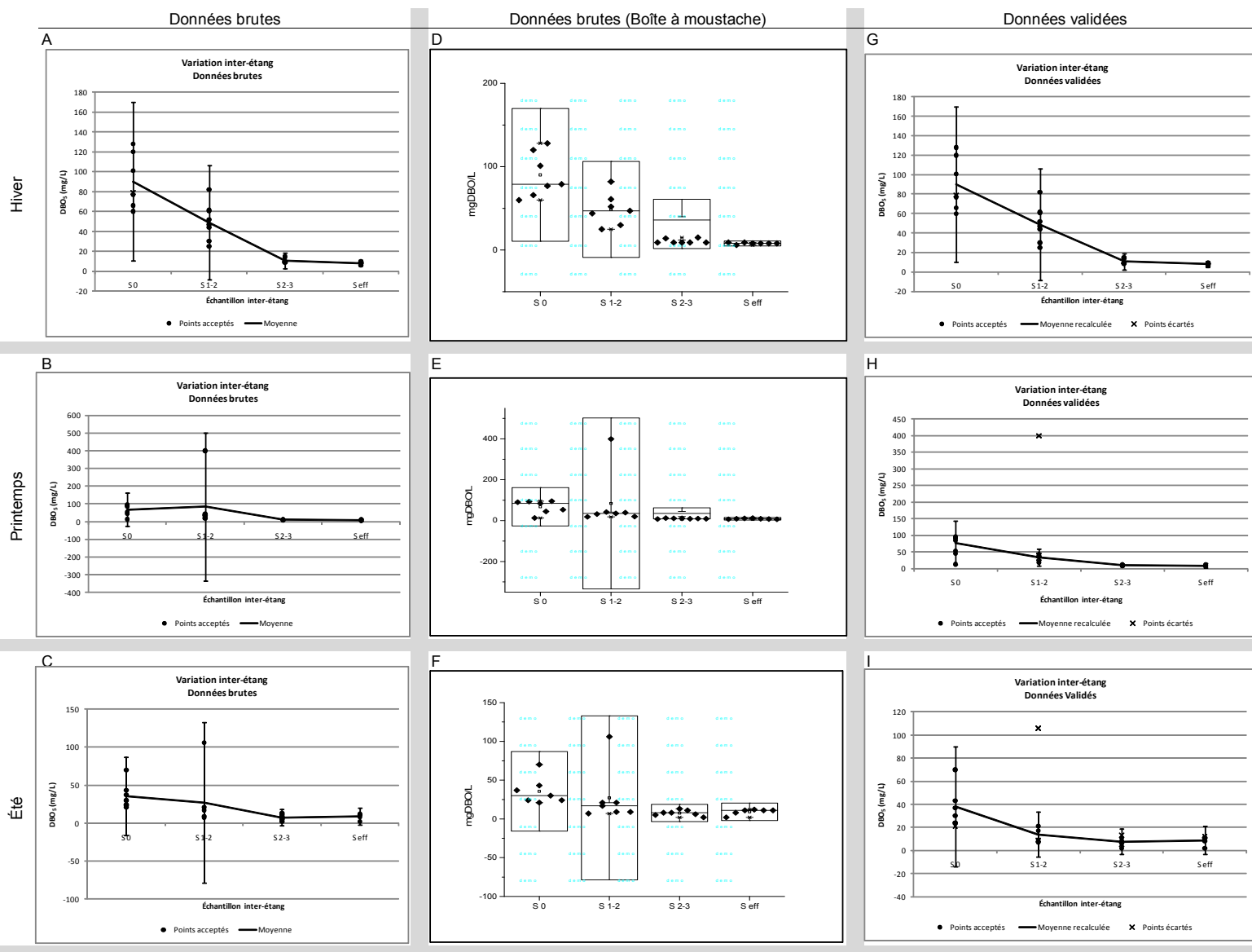
Figure 6.12 : Graphiques de validation des données de DBO 5 de St-Félix-de-Valois
