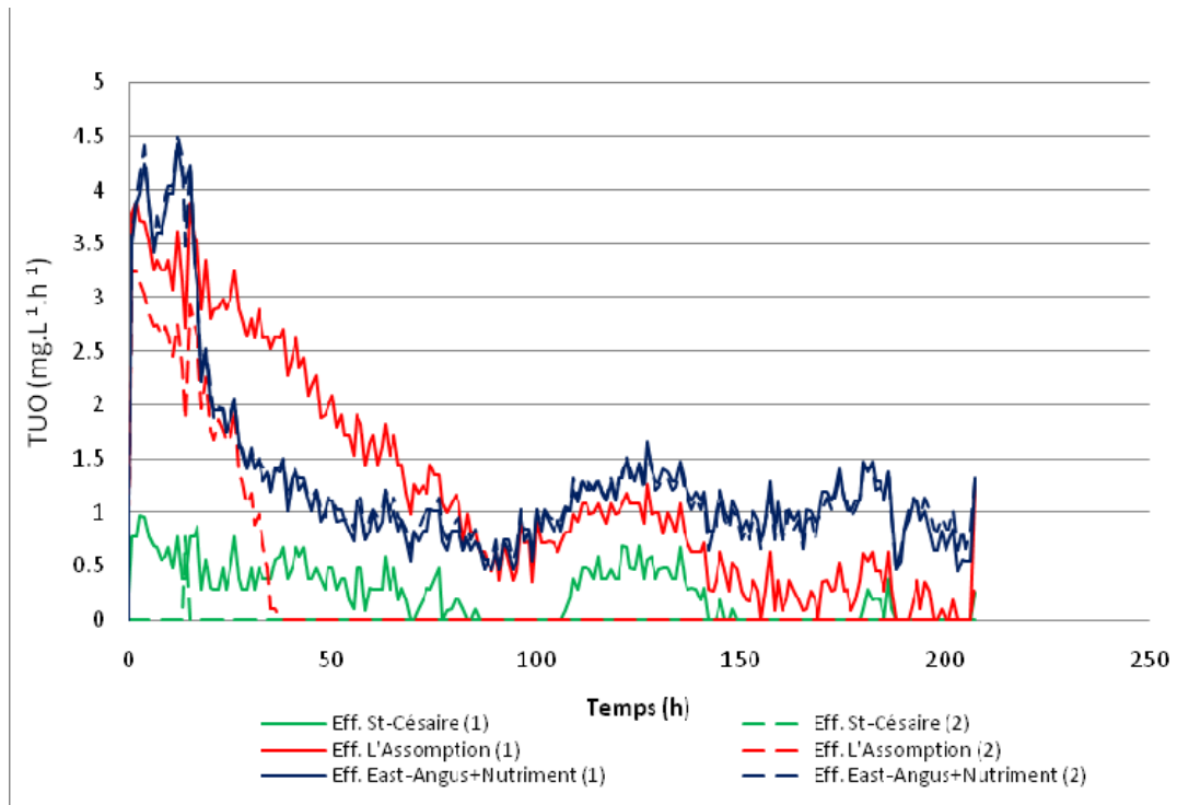
Figure 5.21 : Courbes de respiration endogène pour les échantillons du printemps (jour 2)
