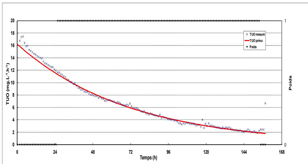
Figure 5.28 : Courbe de respiration endogène de la bouteille 2 de l'effluent de l'Assomption (600 mL) + ATU – Essais d'optimisation n°2
