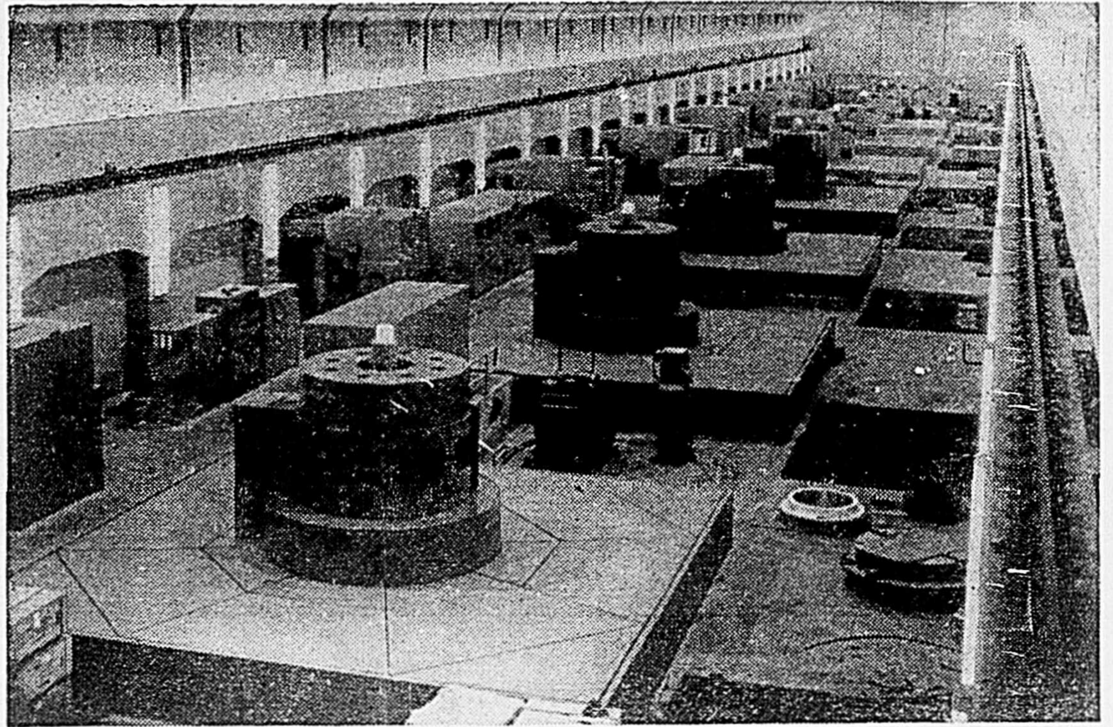
La centrale Bersimis I montrant les huit groupes générateurs, de 150,000 chevaux chacun, raccordés à la ligne de transport reliant Bersimis, Québec et Montréal.
