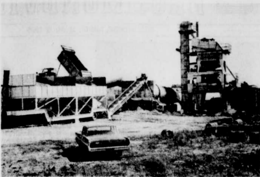
USINE PORTATIVE. — Toute cette usine à asphalte est portable; on peut la démonter et la transporter ailleurs en trois jours.
