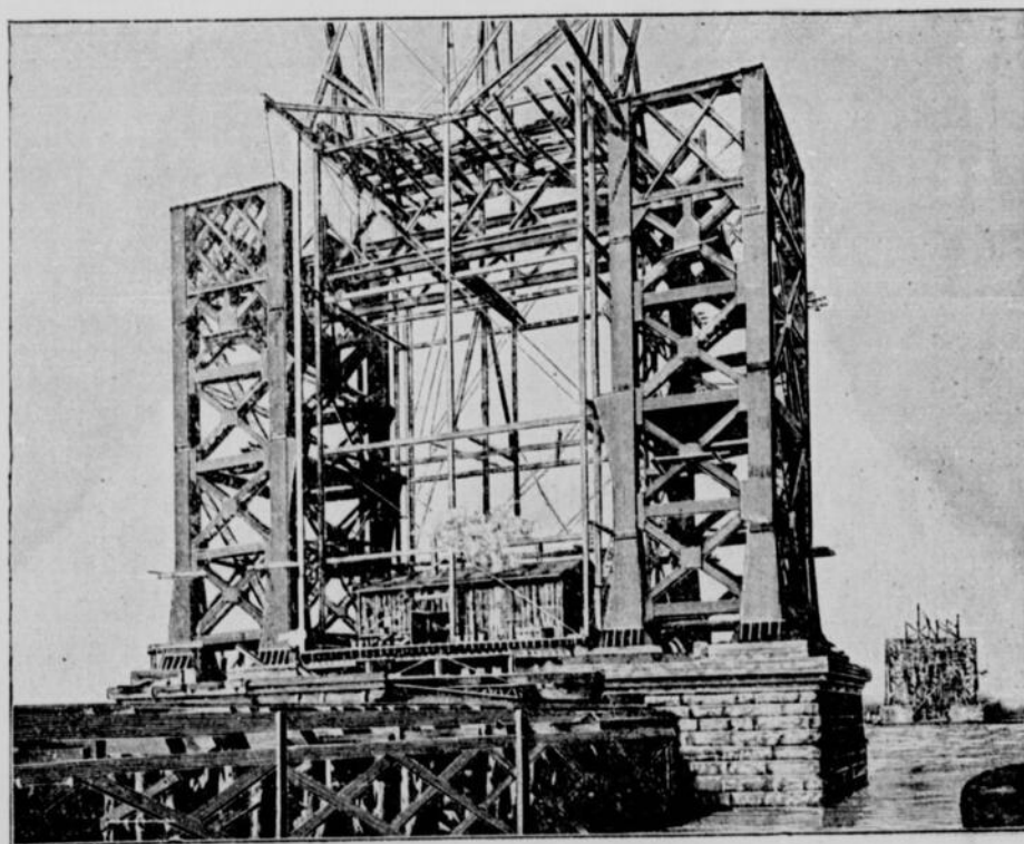
LE NOUVEAU PONT SUSPENDU DE NEW-YORK. — ÉTAT ACTUEL DU MONTAGE DES PIÈCES
