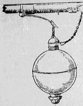
Extincteur Automatique avec déon- tation et signal d'alarme
