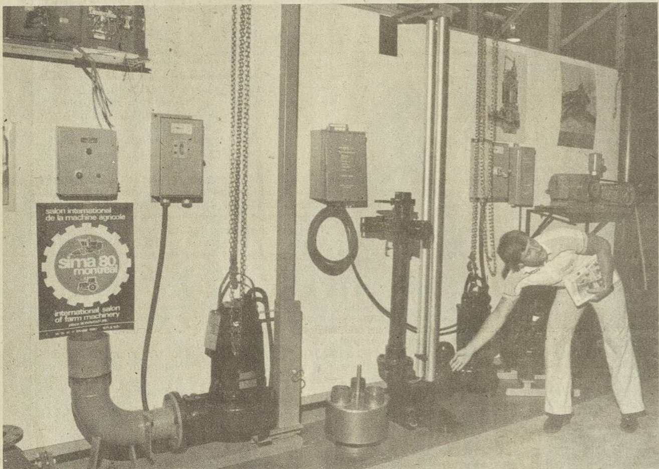
Ces pompes permettent à l'appareil de séparer le liquide du solide dans le purin.
