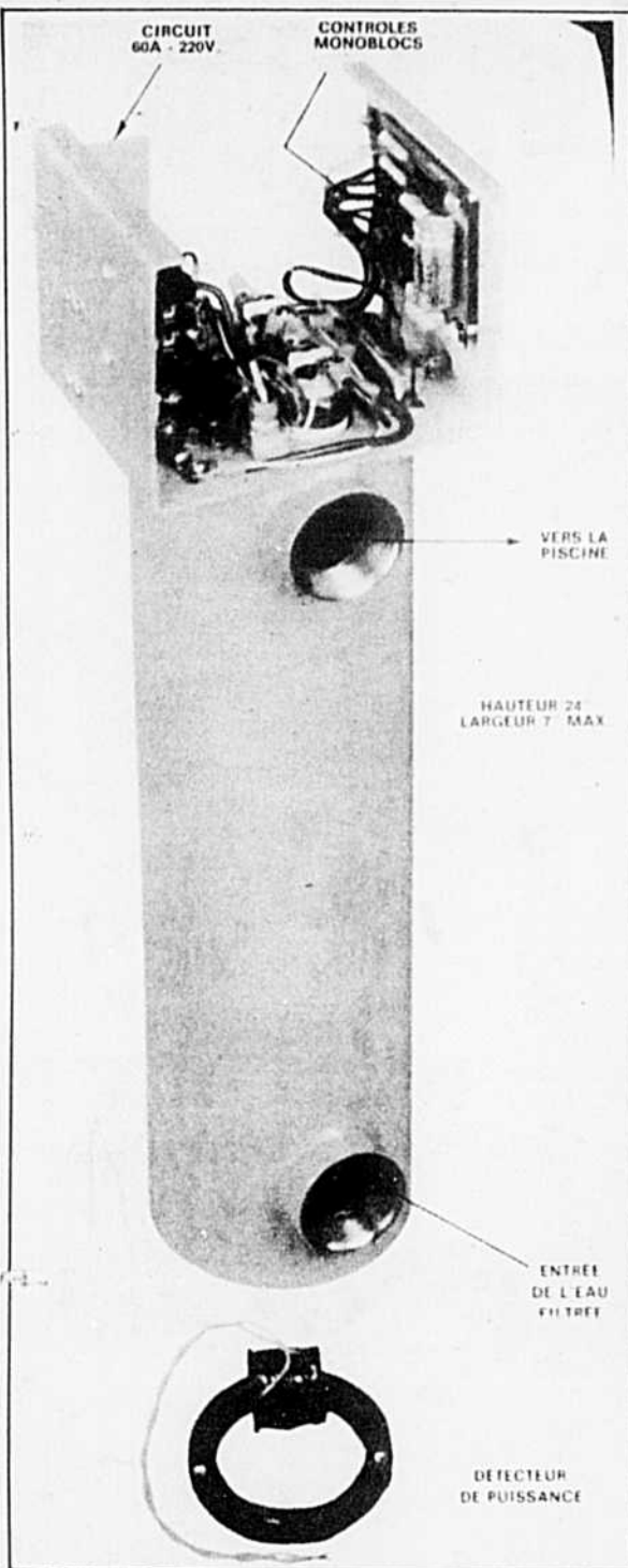
Le chauffe-eau électronique PSC.
