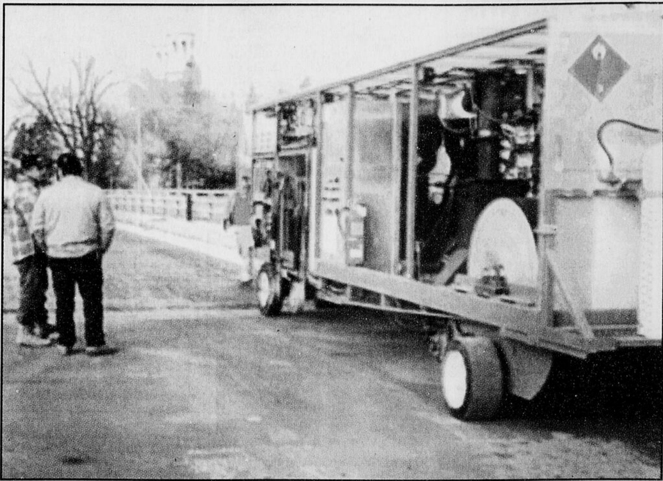
Le Macaden peut appliquer des revêtements comme des membranes d'étanchéité sur des ponts ou des stationnements dans une seule et même opération. Toutes les opérations sont contrôlées par ordinateur, ce qui fait que l'exécution des travaux est à la fois rapide et facile, tout en éliminant les risques de malfaçons.
