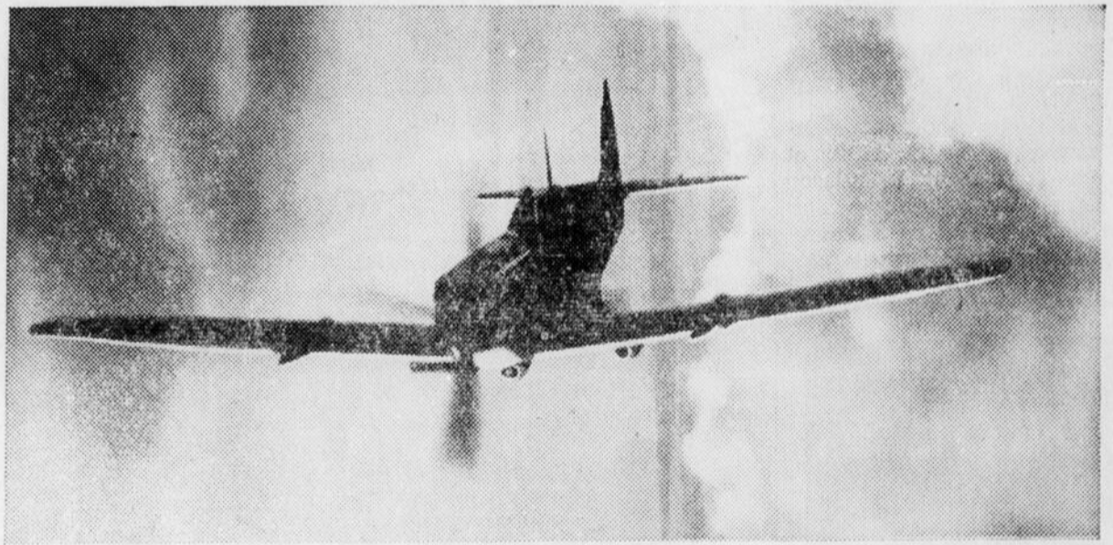
Le Spitfire Mark XII, la version la plus perfectionnée du fameux chasseur de la R.A.F., muni du moteur Rolls Royce Griffon. Les traits saillants de cet avion sont ses ailes abattues qui lui permettent de voler à basse altitude, son nouveau gouvernail effilé et son nez à forme nouvelle qui renferme le moteur Griffon.
