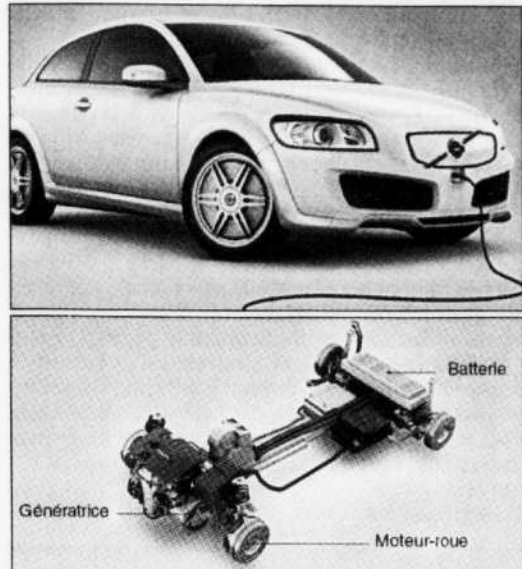
VOLVO Volvo a conçu une voiture équipée de moteurs-roues électriques semblable à celle du physicien hydro-québécois Pierre Couture.
