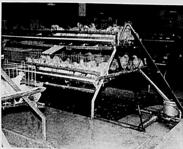
Trois rangées de cages formant triangle permettent aux déjections de tomber directement sur la dalle où elles sont enlevées par le recureur automatique.
