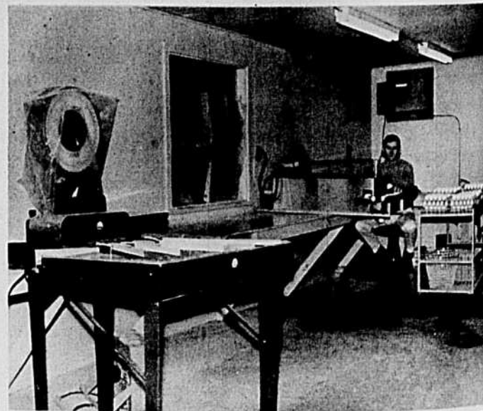
Éleveuse et poulailler sont séparés par la chambre de contrôle, où l'on fait sur les oeufs tous les tests exigés par les expériences en cours.
