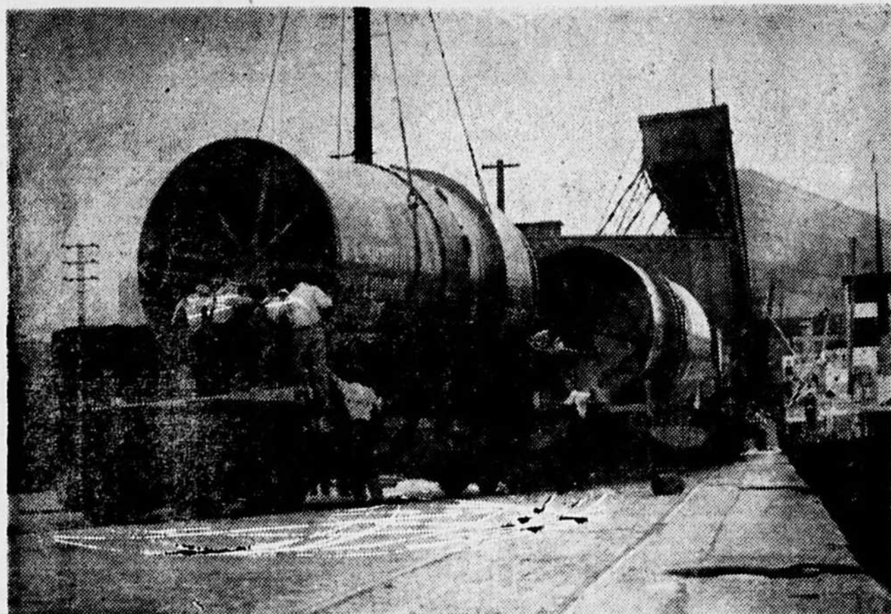
FOUR EXPÉDIE DU R-UNI — Une section du premier four à être expédié au Canada depuis la seconde grande guerre est arrivée à Montréal, mardi venant d'Angleterre. Cette section en acier de 25½ tonnes que l'on est à charger sur un wagon plate-forme du Canadien National mesure 11 pi. de diamètre et 23 pieds de long. Il est adressé à l'usine de la Steelley Company of Canada Ltd., de Dundas, Ont. Le four servira à produire du dolomite, produit utilisé dans la réparation des fours et des fournaies électriques. (Photo Canadien National.)
