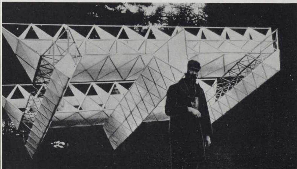
Un menuisier de Beinn Bhreagh tire un cerf-volant tétraédrique du Dr Bell (photographie prise en 1902). Ce modèle, solide mais léger, s'élevait bien au-dessus de la terre, mais on constata qu'on ne pouvait le manoeuvrer à l'aide de moteurs.
