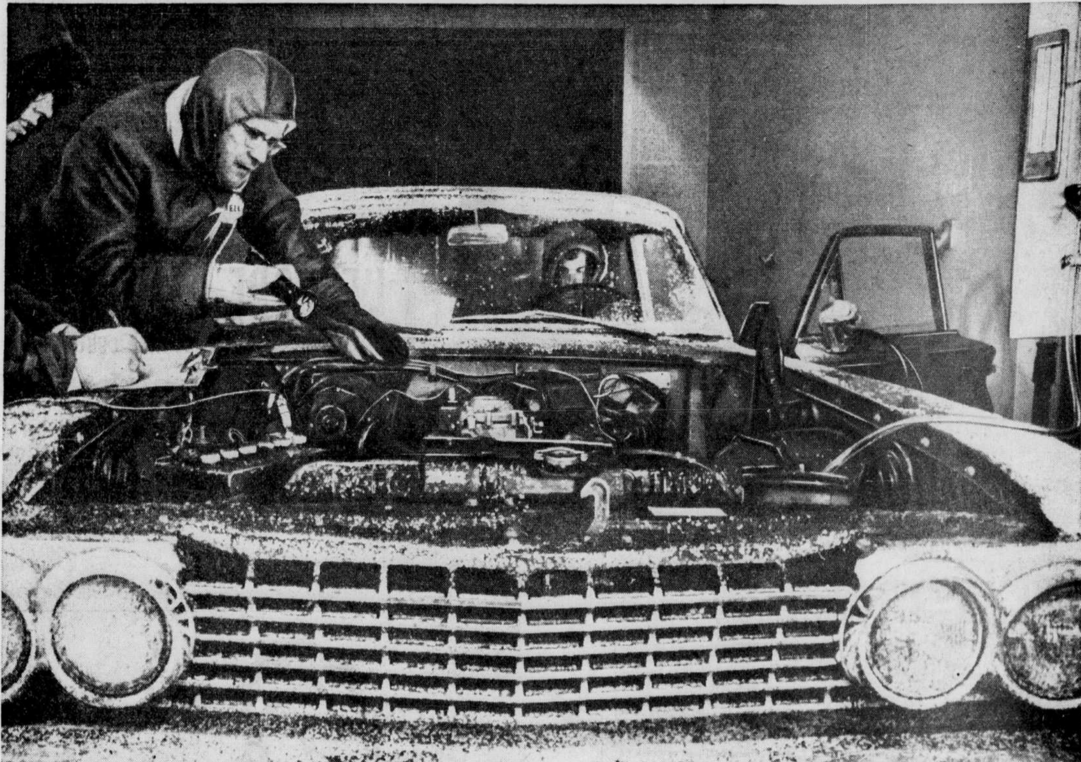
Les techniciens de Shell mettent aux essais de performance, dans leur nouveau laboratoire, le Mélange-Hiver spécial de Super Shell. La température est de 40 au dessous de zéro.
