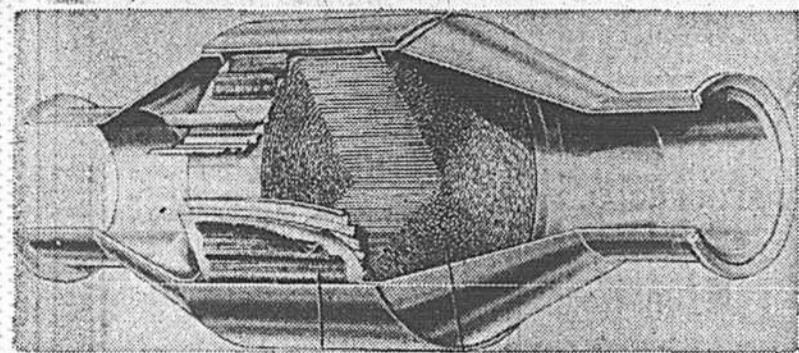
Au cœur du problème technique actuellement posé par "l'épuration" de l'automobile, le convertisseur catalytique, dispositif placé dans le circuit d'échappement, qui achève la combustion des gaz nocifs qui n'ont pas été entièrement consommés dans les cylindres du moteur. Il s'agit ici du modèle en nid d'abeilles de Ford.
