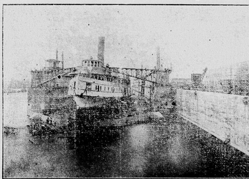
Vue de la Cale-sèche flottante à Montréal, avec bateau en réparation
