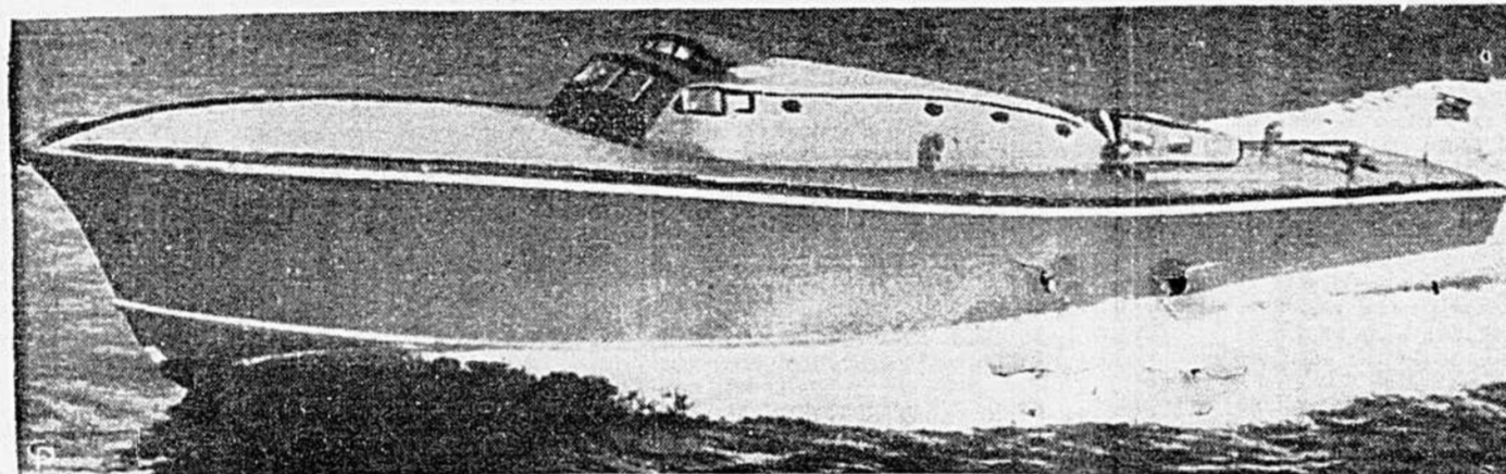
Au large de l'île de Wight, près des côtes d'Angleterre, les ingénieurs de la marine britannique ont effectué, avec succès, les essais nautiques de ce petit torpilleur. Voici les caractéristiques de ce nouveau vaisseau de guerre dont plusieurs unités sont actuellement en construction: Vitesse, 50 milles à l'heure, propulsée par 3 moteurs de 1,000 chevaux-vapeur; armement: 2 tubes lance-torpilles de 21 pouces ou 4 tubes de 18 pouces. Le navire est long de 70 pieds, sans mât ni cheminée, ce qui fait qu'il est une cible difficile à atteindre si on tient aussi compte de sa rapidité.
